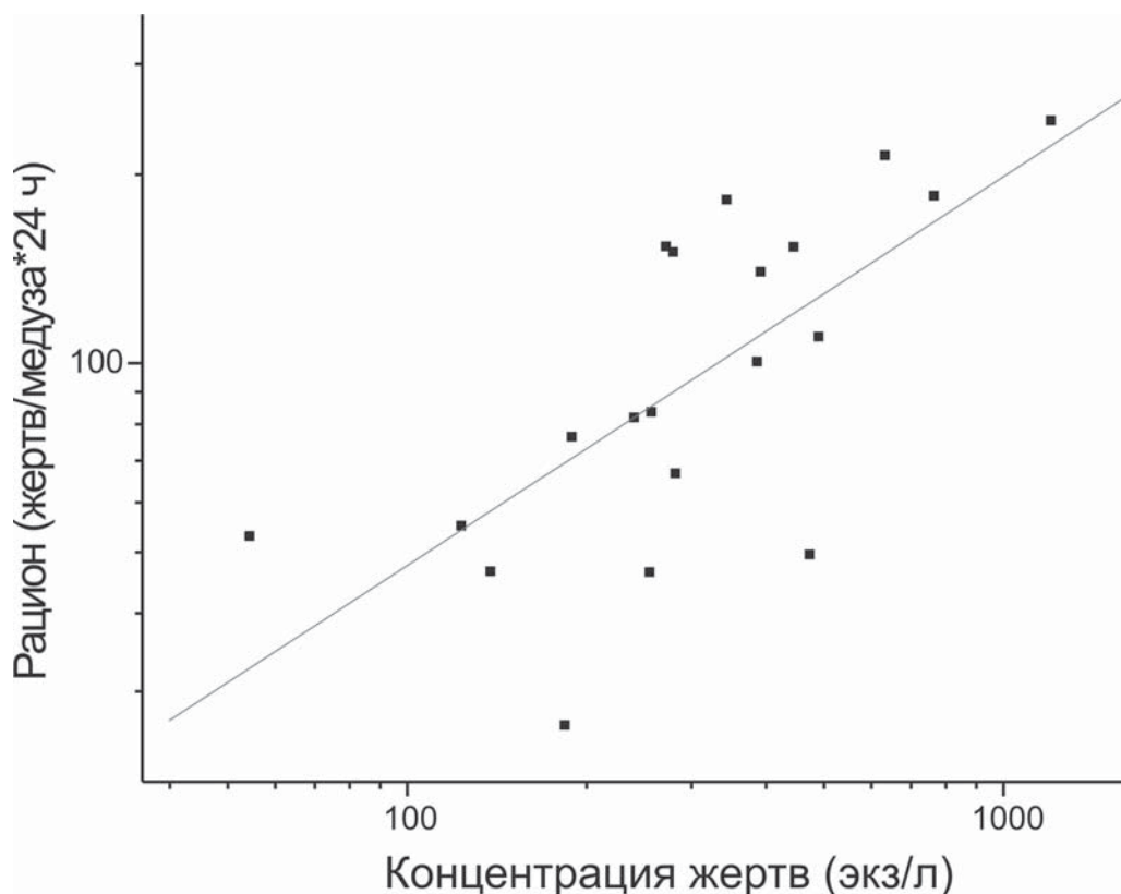
Рис. 4. Зависимость суточного потребления жертв медузами Bougainvillia superciliaris от концентрации зоопланктона.
